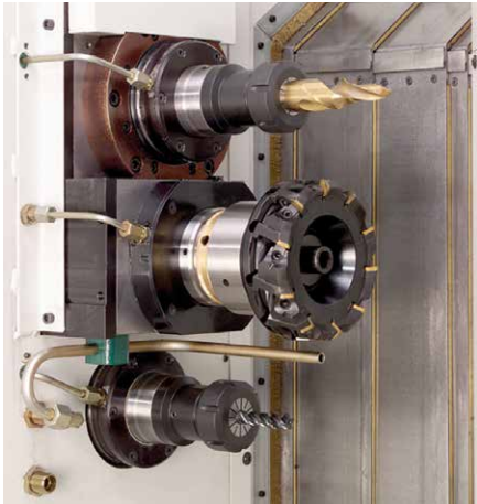
Bearbeitungseinheiten mit 1, 2 oder 3 Spindeln
